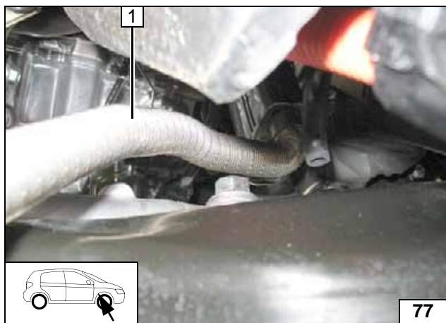
1 Abgasendstück
