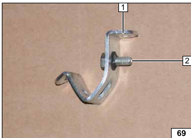
1 Lochband 2 Schraube M6x16, Bolzensicherung
