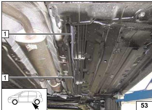
1 Wellrohr 2100 mit Brennstoffleitung und Kabelbaum Dosierpumpe
