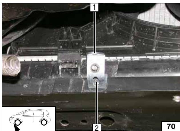
1 Lochband 2 Schraube M6x20, Federring, vor- handene Gewindebohrung
