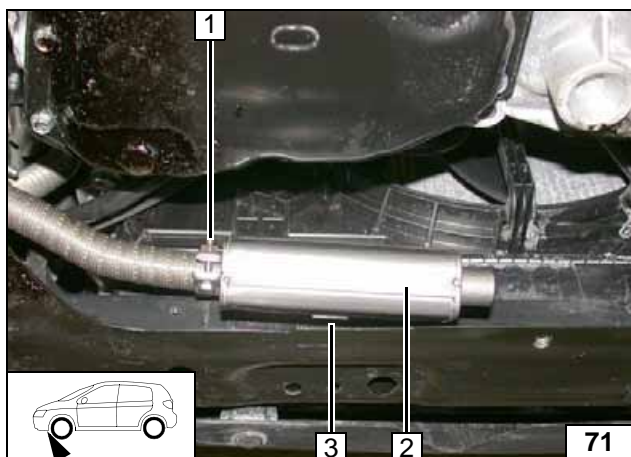
Schalldämpfer 2 mit vormontierter Schraube M6x16 an Lochband 3 befestigen. Schalld- dämpfer 2 ausrichten, ggfs. nachbiegen!
