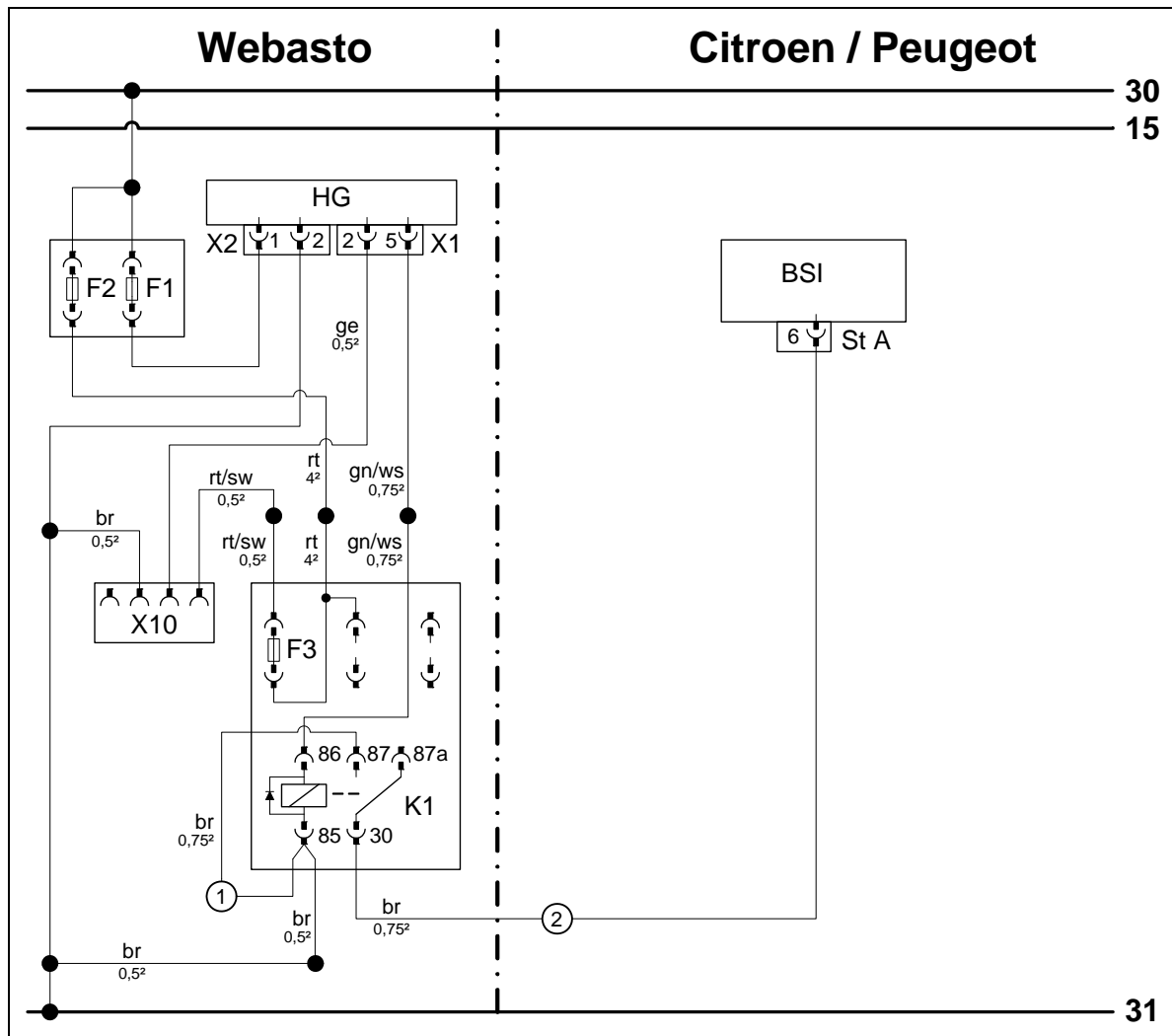
Schaltplan
