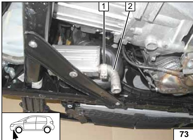
1 Schlauchklemme 2 Abgasendstück
