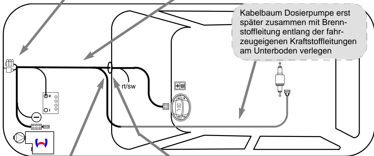
Schema Kabelbaumverlegung
