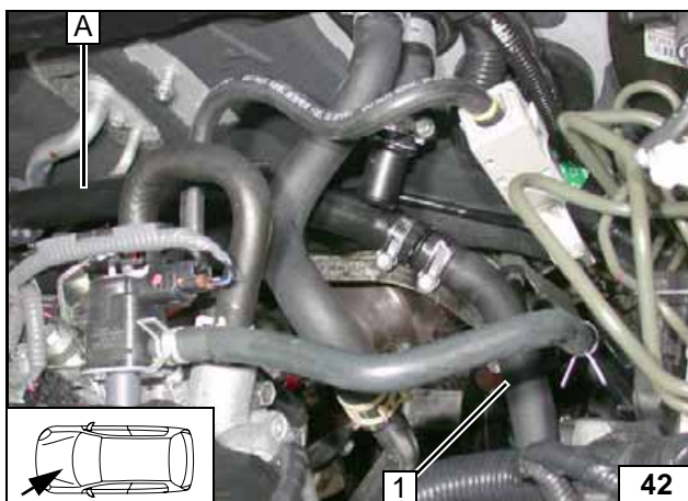
1 Schlauchstück Motoraustritt
