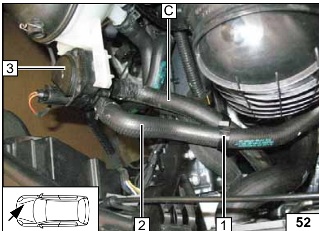
3 Fahrzeugeigene Umwälzpumpe
