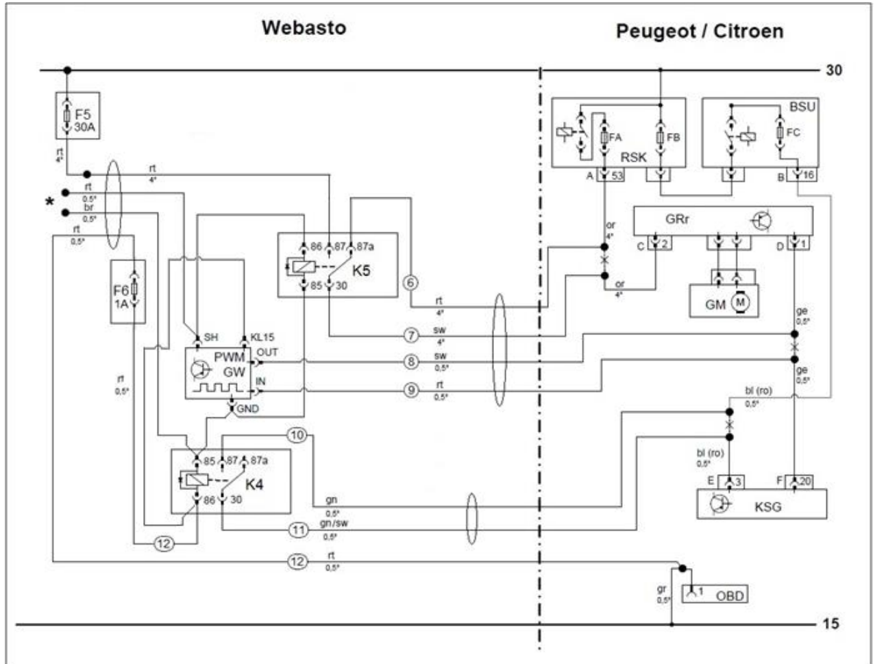
Принципиальная схема
