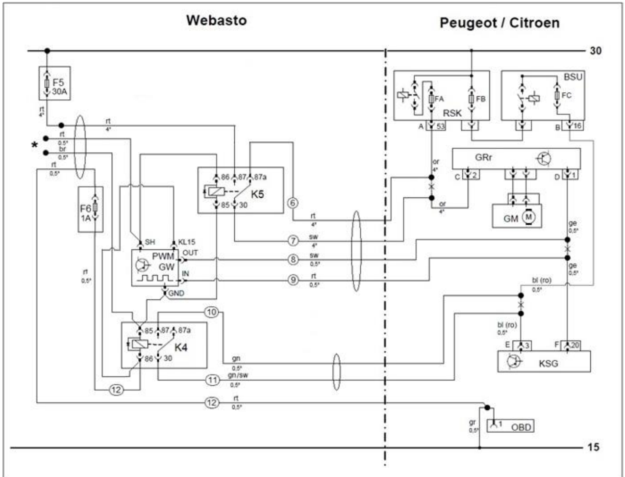
Принципиальная схема
