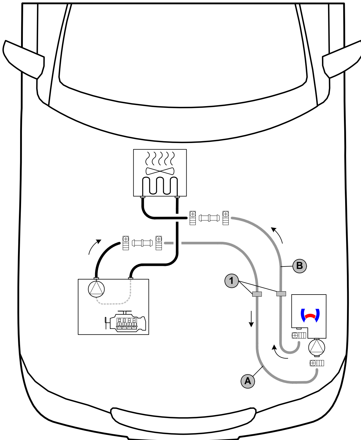
Schema Wasserverlegung
