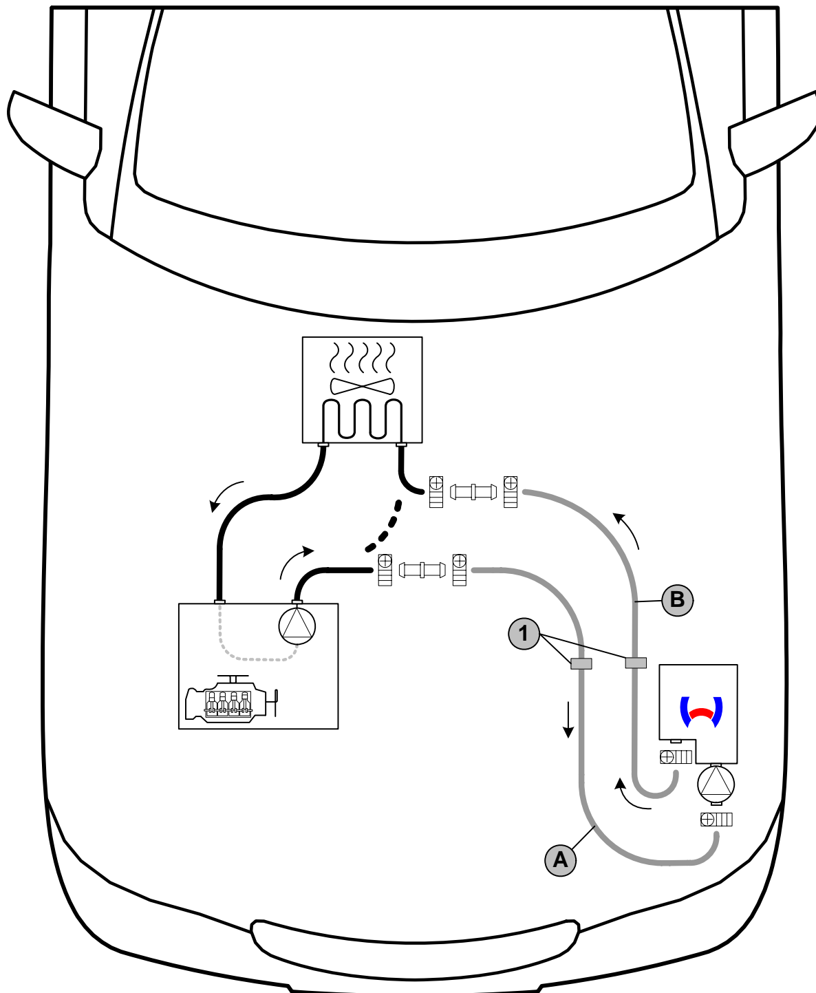
Schema Wasserverlegung
