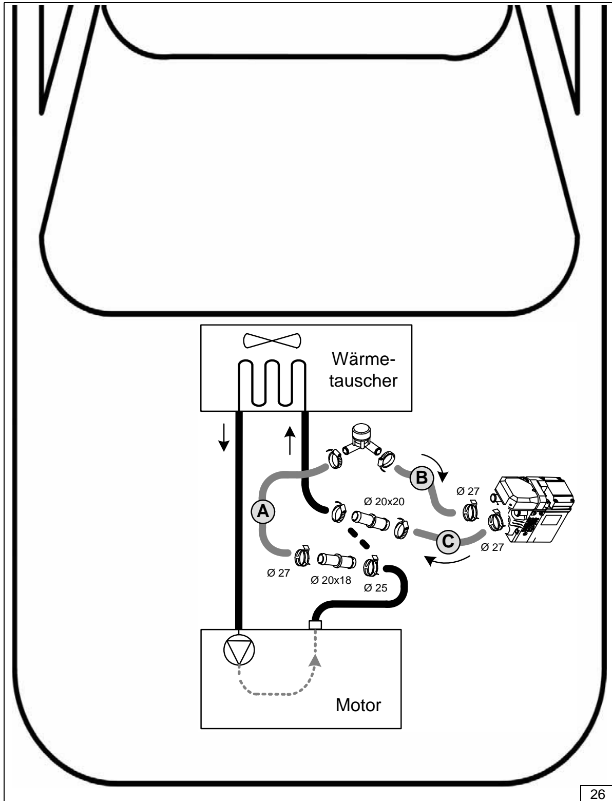
Schema Wasser
