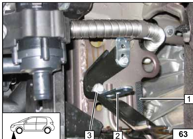
1 Kantenschutz 50 2 Vormontiertes Lochband 3 Fzg.eigene Schraube
