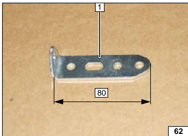
Lochband 1 um 90° abwinkeln.
