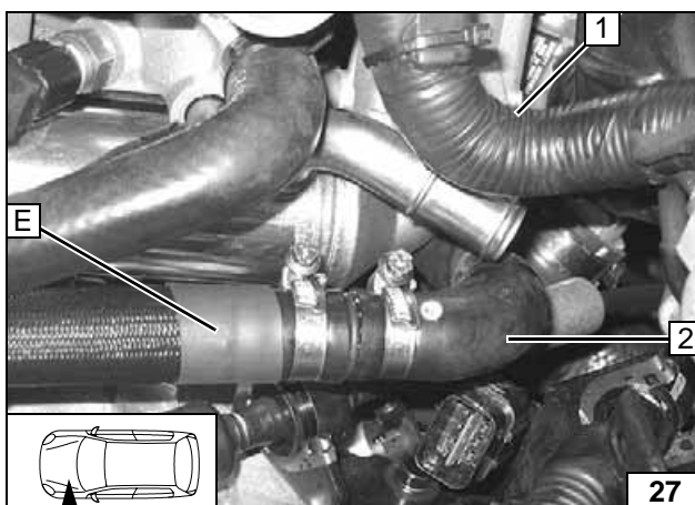
2 Schlauch Wärmetauschereingang
