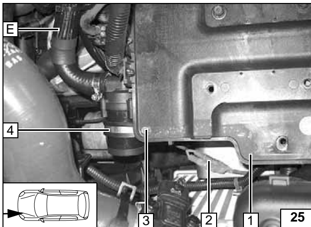
4 Umwälzpumpe, gummierte Rohrschelle Ø 48mm, Schraube M6x20, Bundmutter
