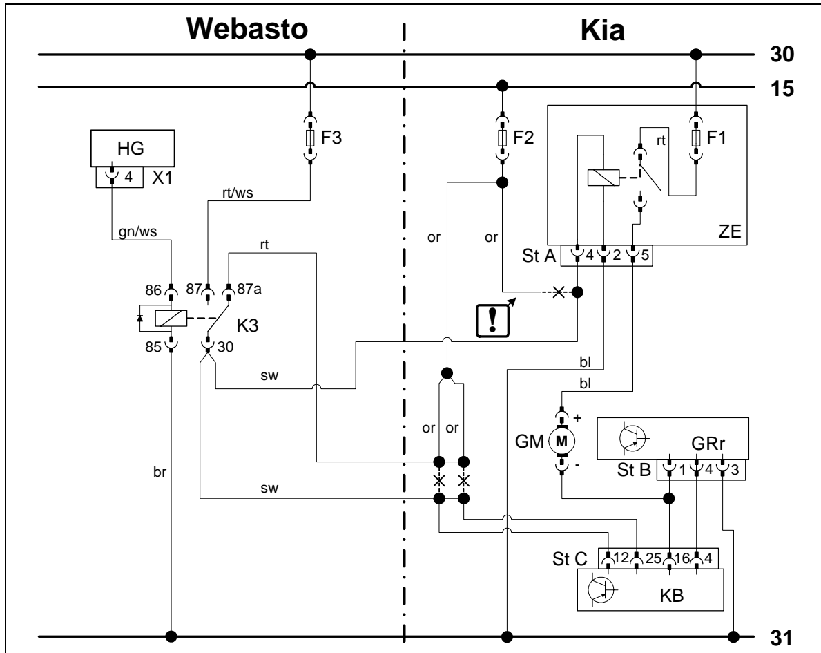
Schaltplan Klimaautomatik
