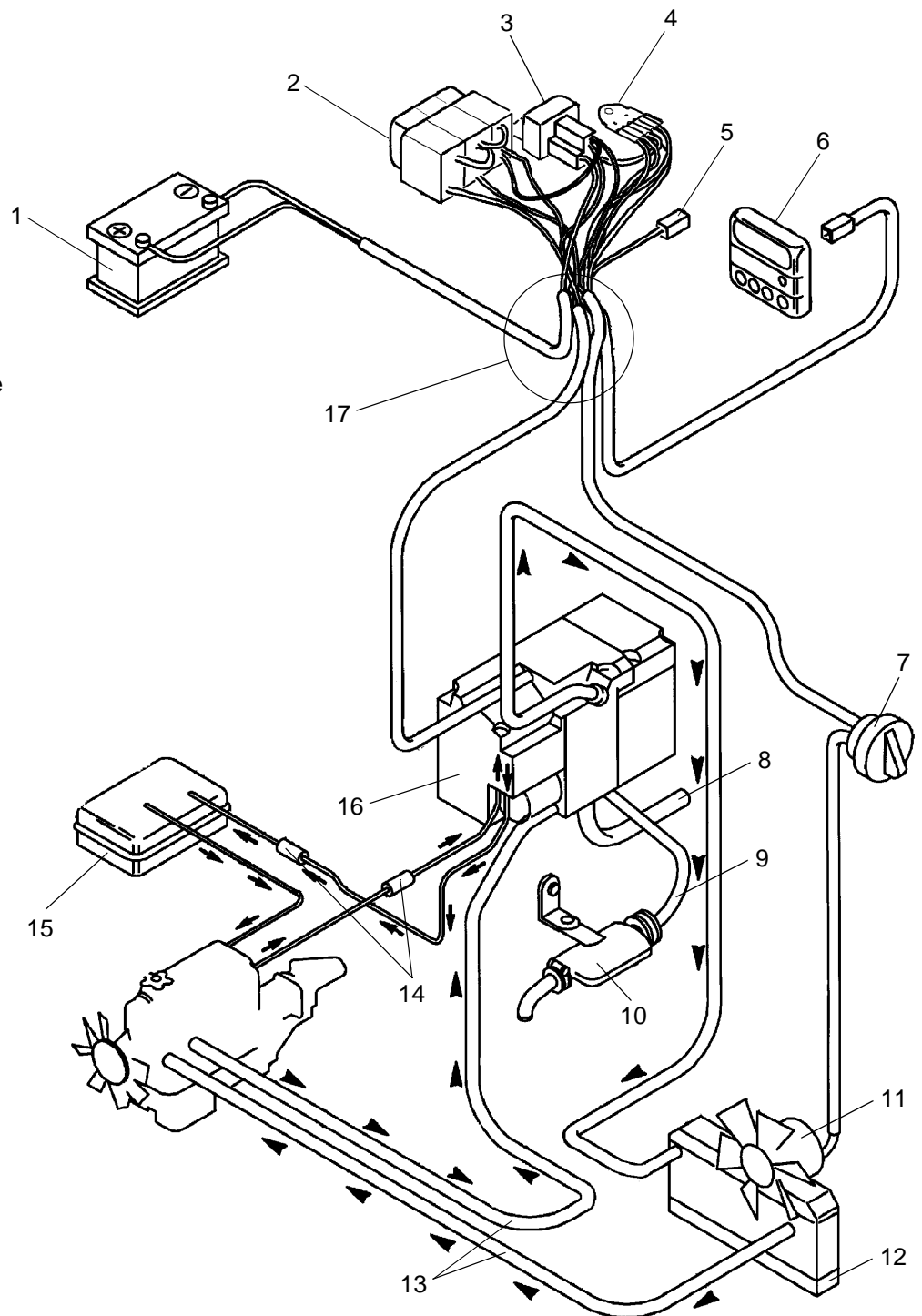
Abb. 501 Repräsentative Einbauanordnung im Fahrzeug
