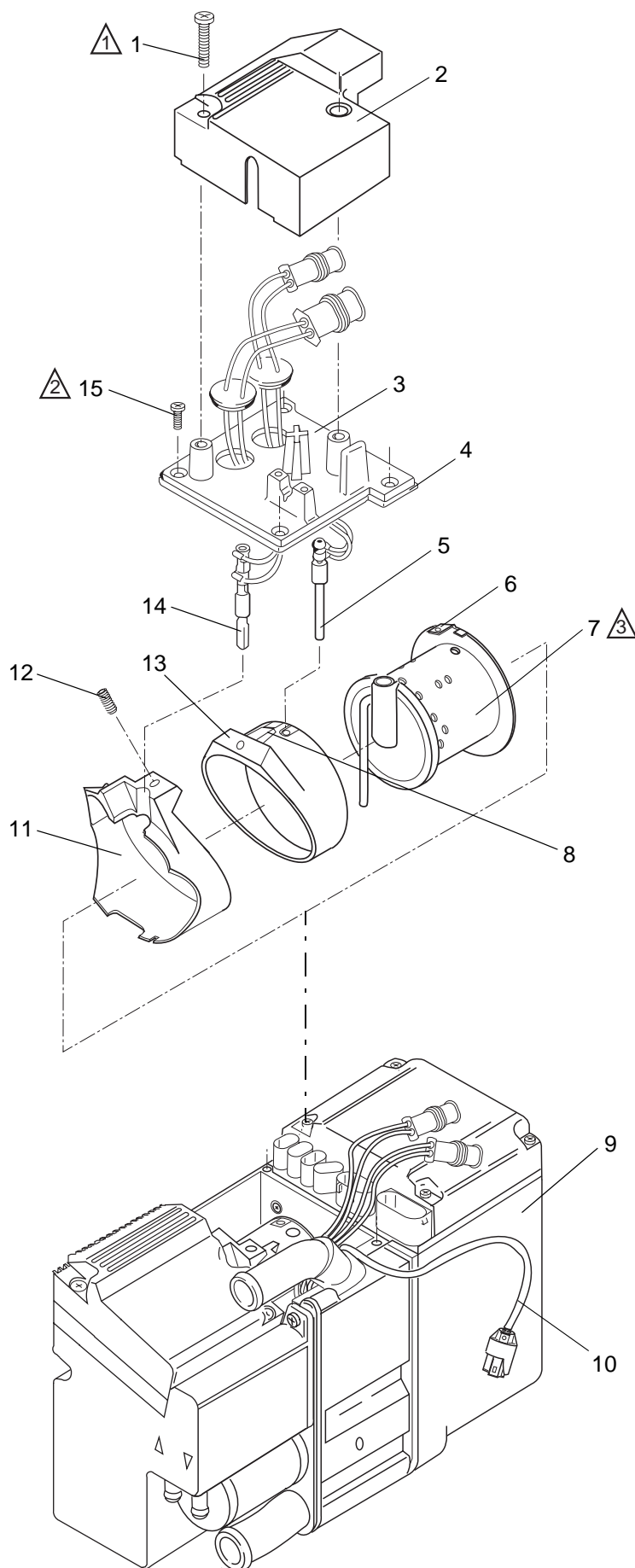
Abb. 809 Wechsel des Brenneinsatzes (Seite 1 von 2)
