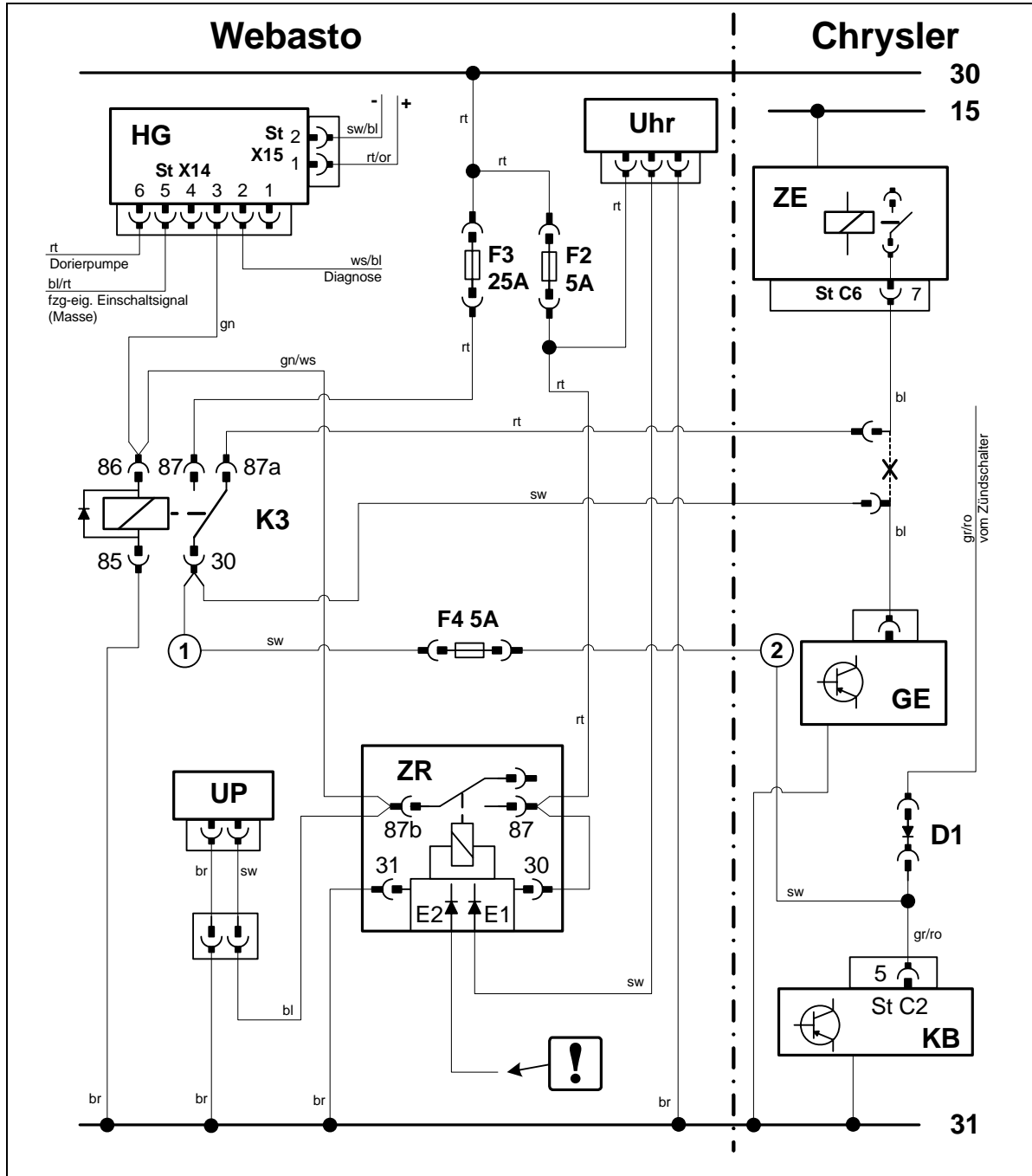
Schaltplan 2-Zonen- und 3-Zonen- Klimauto- matik
